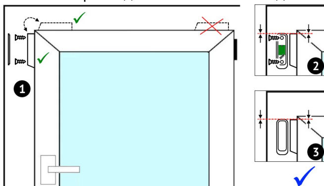
Малюнок 2. Встановлення з відкриванням ліворуч
